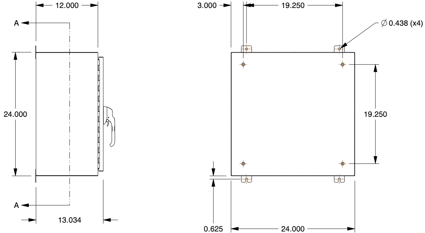
SECTION A-A
