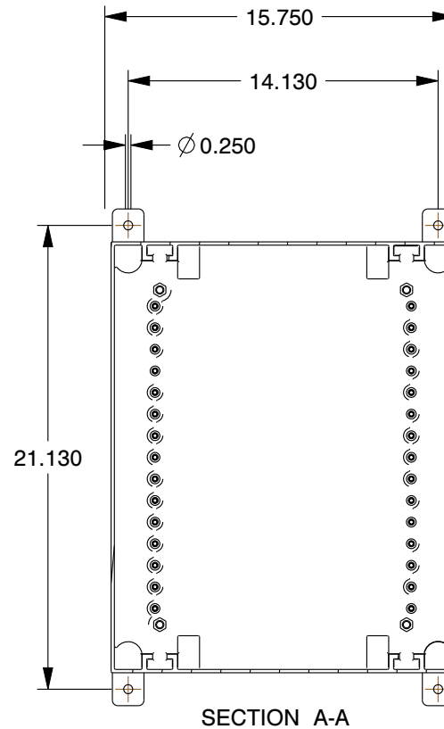
SECTION A-A
