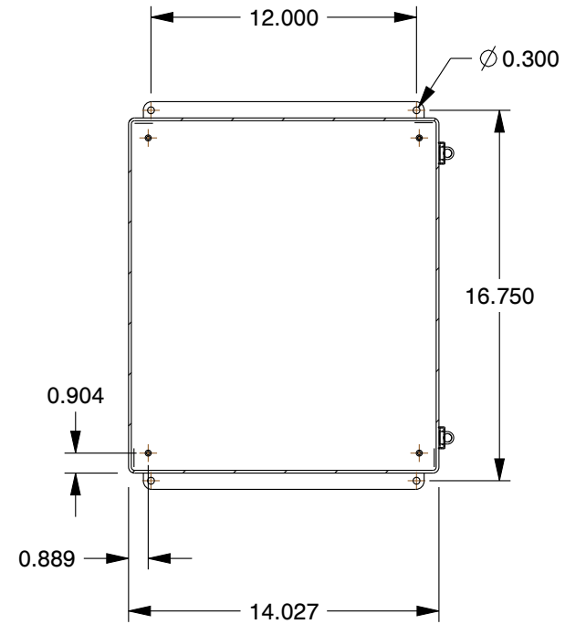
SECTION A-A
