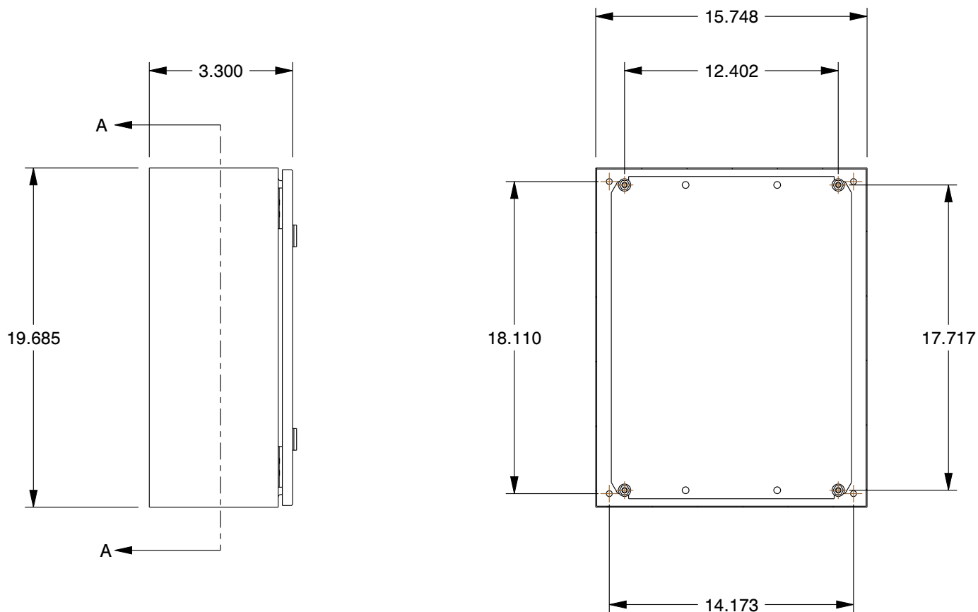
SECTION A-A
