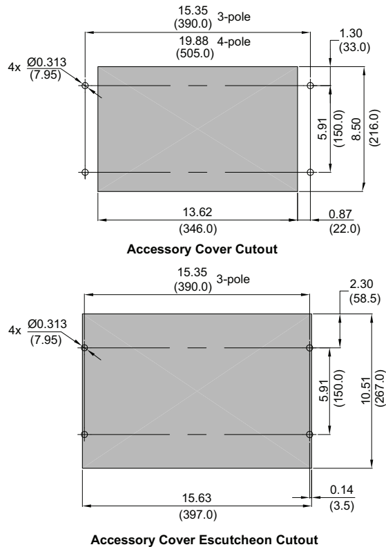
FIG. 2 : Mounting Hole and Enclosure Cover Cutouts Dimensions / Dimensiones de los agujeros de montaje y de los cortes de la cubierta del gabinete / Dimensions des trous de montage et des découpages de couvercle du coffret
