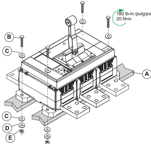
TABL. 2 : Individually-Mounted Circuit Breaker Connections / Conexiones de interruptores automáticos de montaje individual / Montage individuel des connexions de disjoncteur
