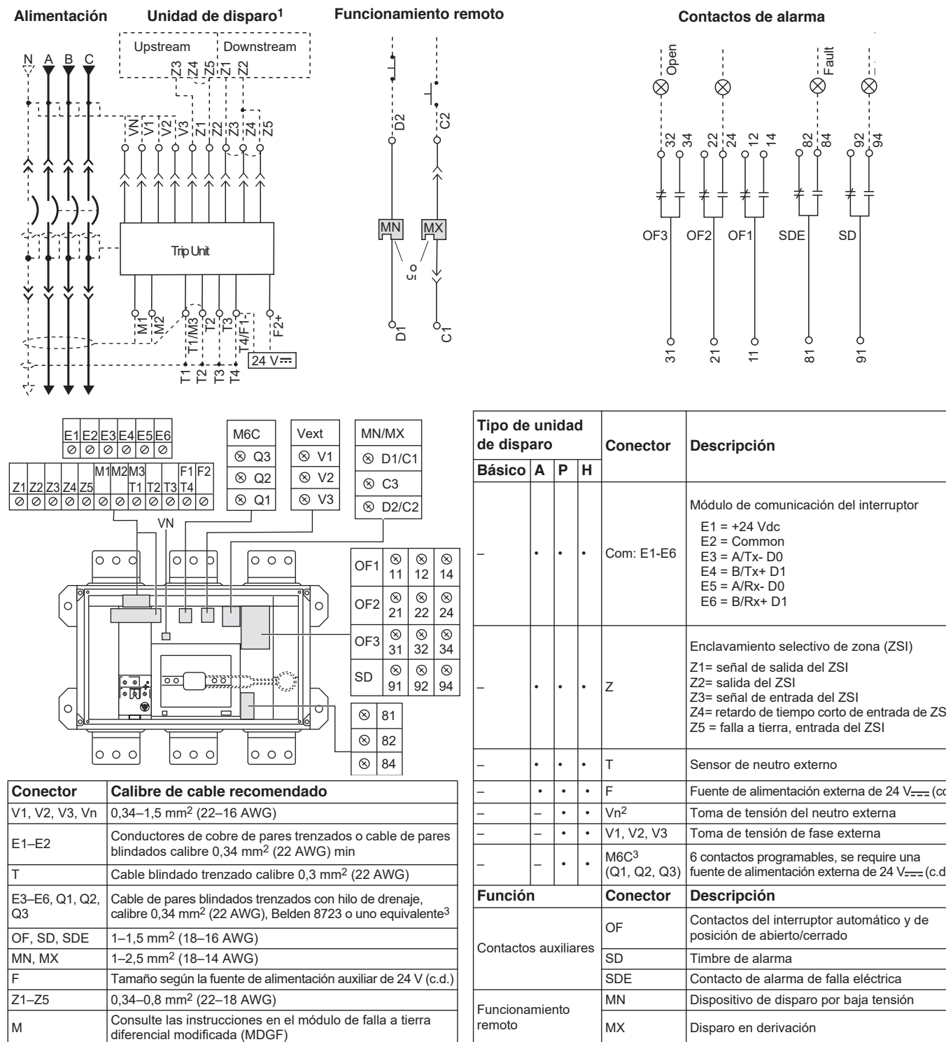
FIG. 4 : Diagramas del cableado de control de los accesorios (Espanol)
