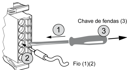
Bloco de terminal
