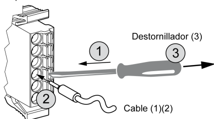
Bloque de terminales
