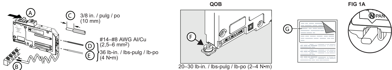
FIG. 1 : Installation / Instalación / Installation
