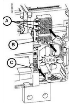
R-frame and NS1600b-NS3200 Circuit Breakers Interruptores automáticos marco R y NS1600b-NS3200 Disjoncteurs à châssis R et NS1600-NS3200 R 型断路器和 NS1600b-NS3200 断路器
