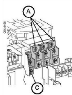
Electrically-operated P-frame and NS630b-NS1600 Circuit Breakers Interruptores automáticos marco P y NS630b-NS1600, de funcionamiento eléctrico Disjoncteurs à commande électrique, à châssis P et NS630b-NS1600 电动操作的 P 型断路器和 NS630b-NS1600 断路器
