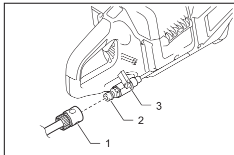
► 1. Manguito del acoplamiento 2. Entrada para agua 3. Llave
