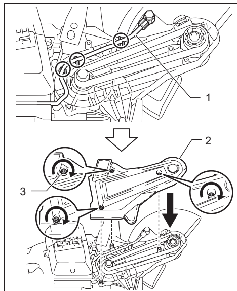
► 1. Tube 2. Cover 3. Hex socket bolt
