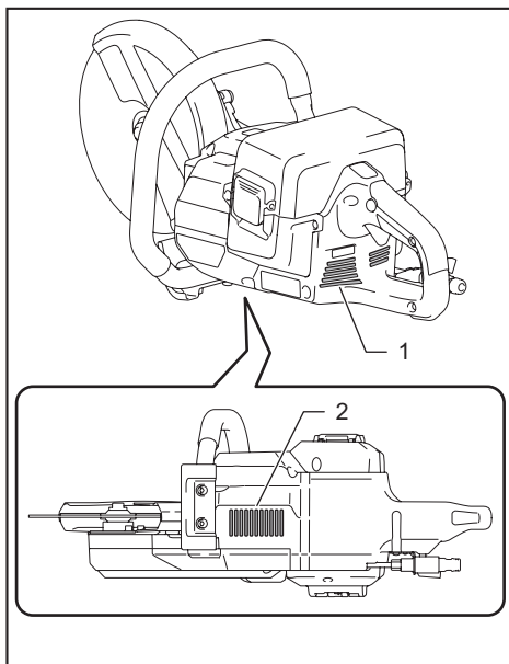
► 1. Ventilación de entrada 2. Ventilación de salida
