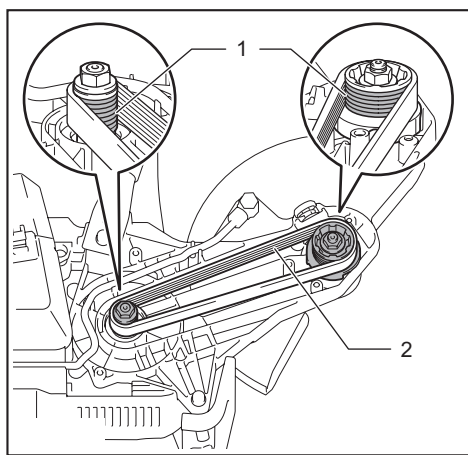
► 1. Riel sobre la polea 2. Guía sobre la correa en V
