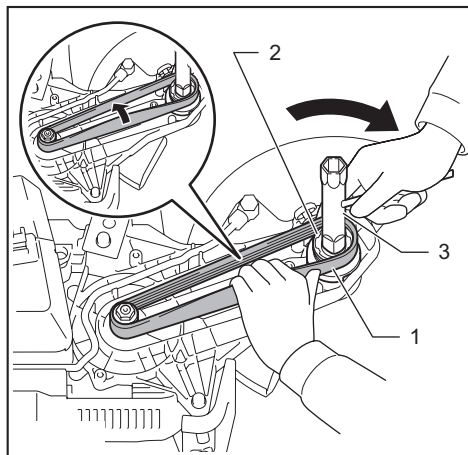
► 1. Correa en V 2. Polea (grande) 3. Llave de ojo
