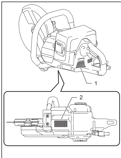
► 1. Inhalation vent 2. Exhaust vent
