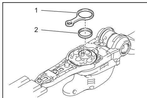
► 1. Rod 2. Bearing
