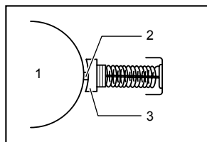
1. Commutateur 2. Bout isolateur 3. Charbon
