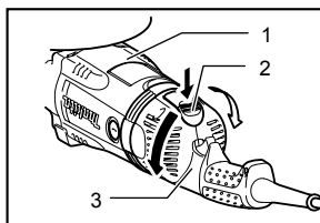
1. Alojamiento del motor 2. Botón de bloqueo 3. Mango
