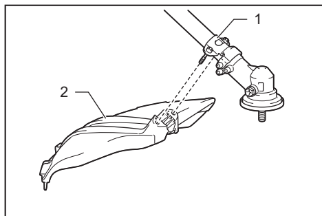
► 1. Clamp 2. Protector
