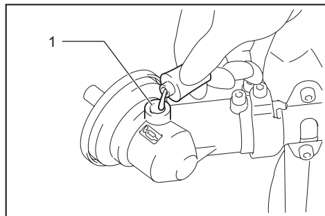
► 1. Orificio para el engrasado
