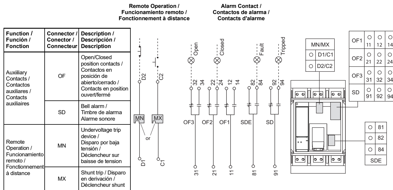
FIG. 3 : Accessory Control Wiring Diagrams / Diagramas del alambrado de control de los accesorios / Schémas de câblage de contrôle des accessoires
