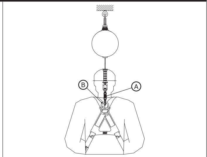
図8 - ハーネスへの接続
