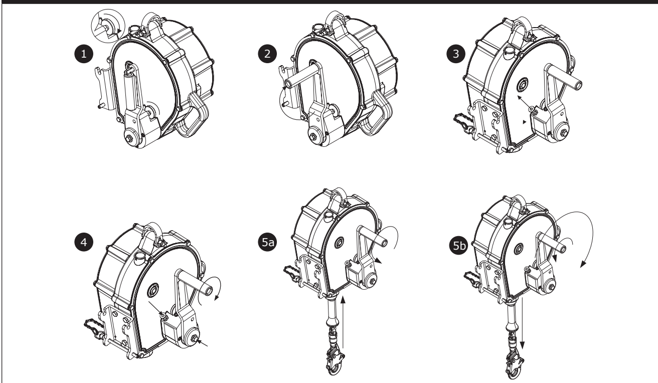
図10 - 巻取り操作
