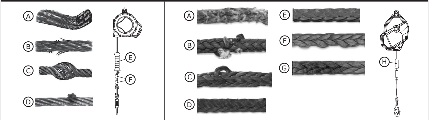
図14 - ワイヤロープ
