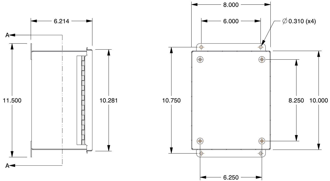
SECTION A-A
