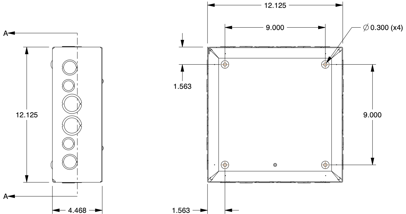
SECTION A-A
