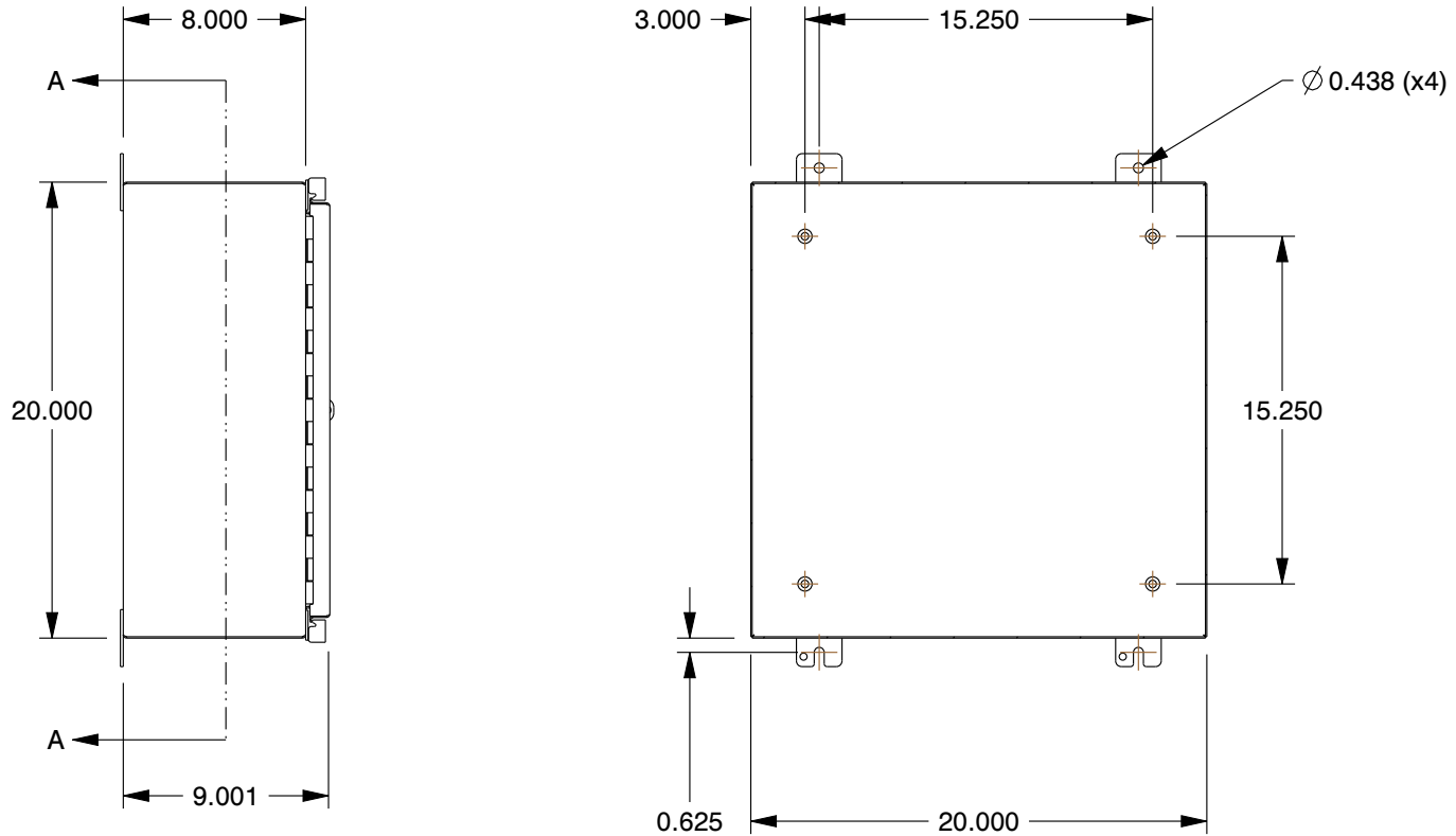
SECTION A-A
