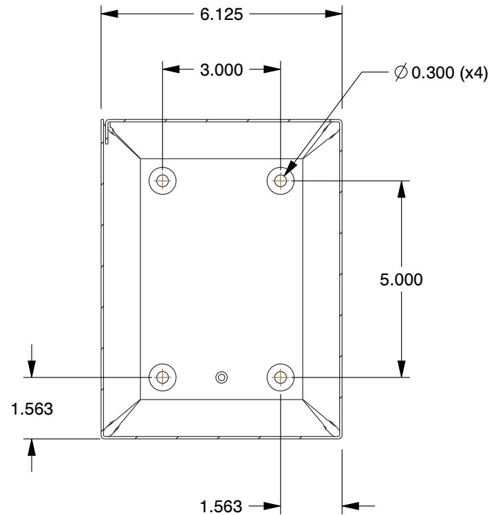
SECTION A-A
