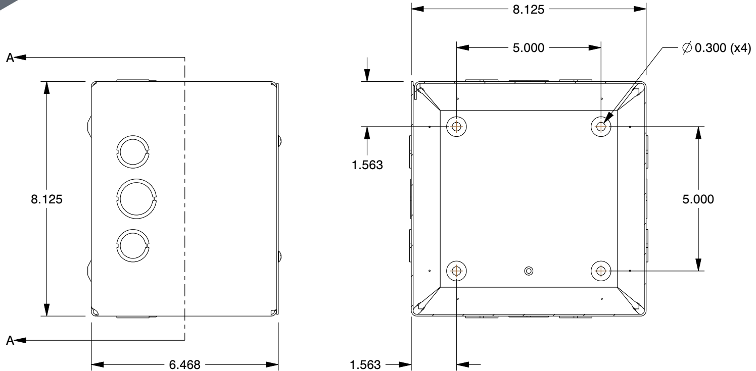
SECTION A-A
