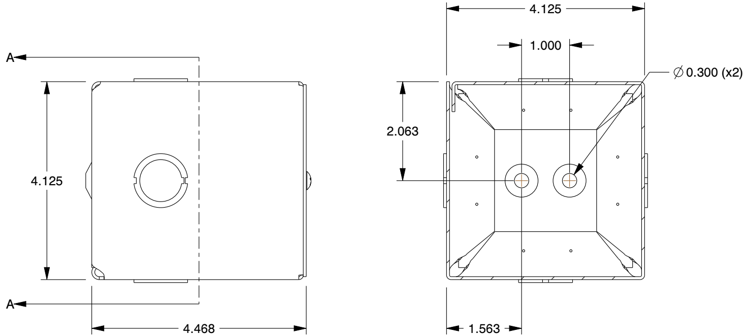
SECTION A-A
