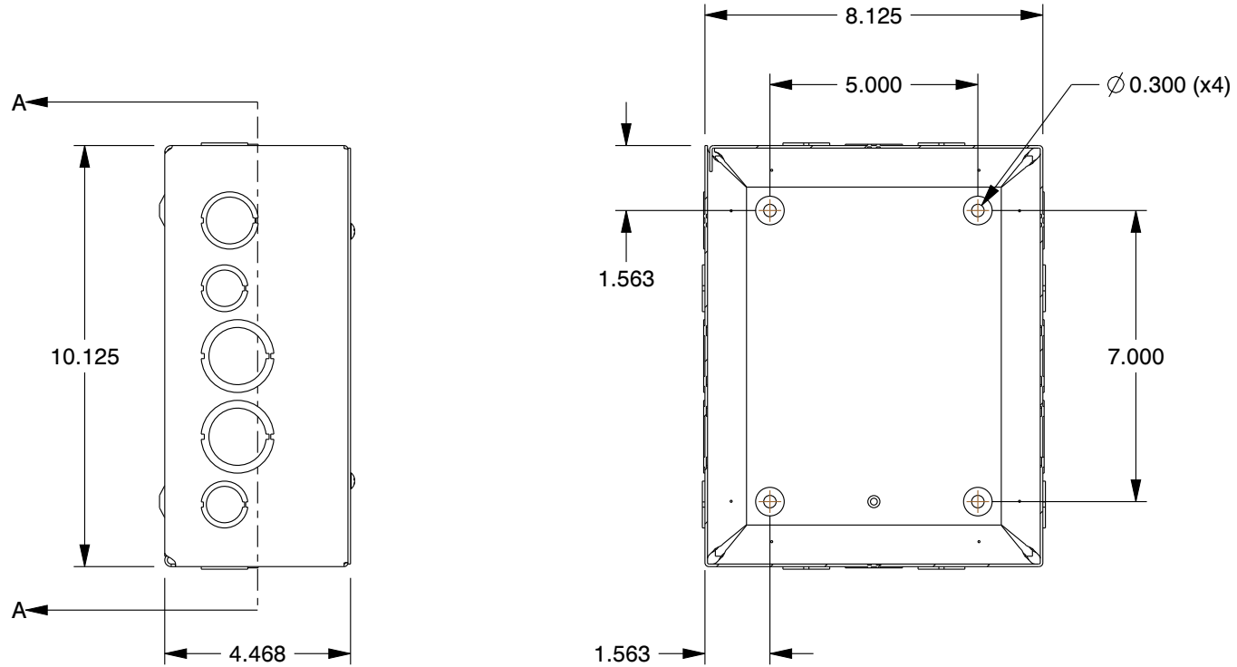
SECTION A-A
