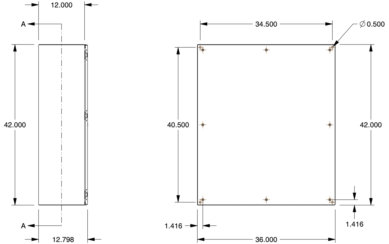
SECTION A-A
