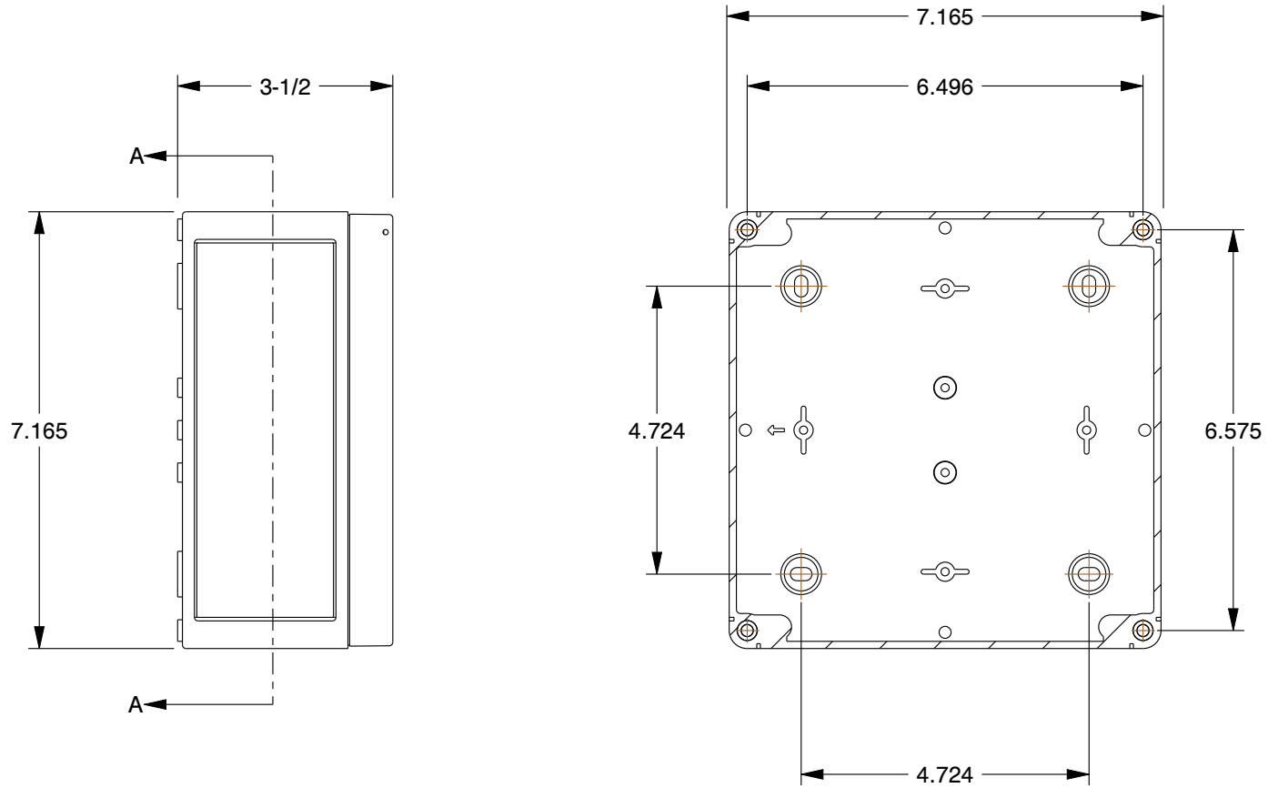
SECTION A-A
