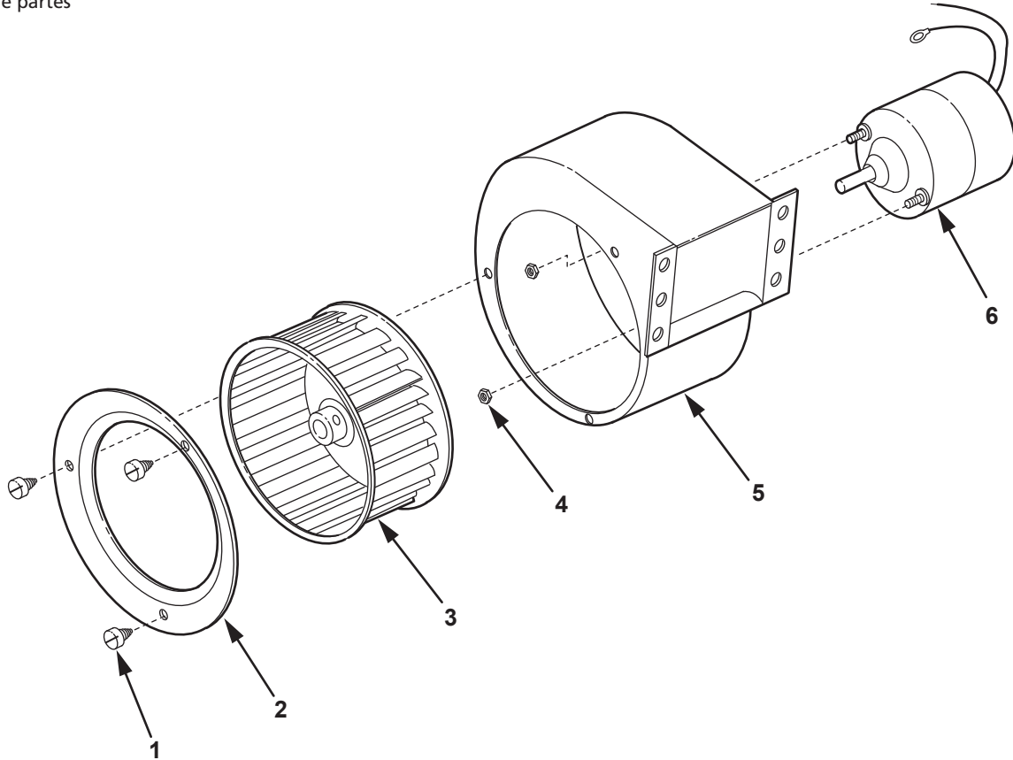
Figura 5 – Ilustración de las Partes de Reparación para los Sopladores
