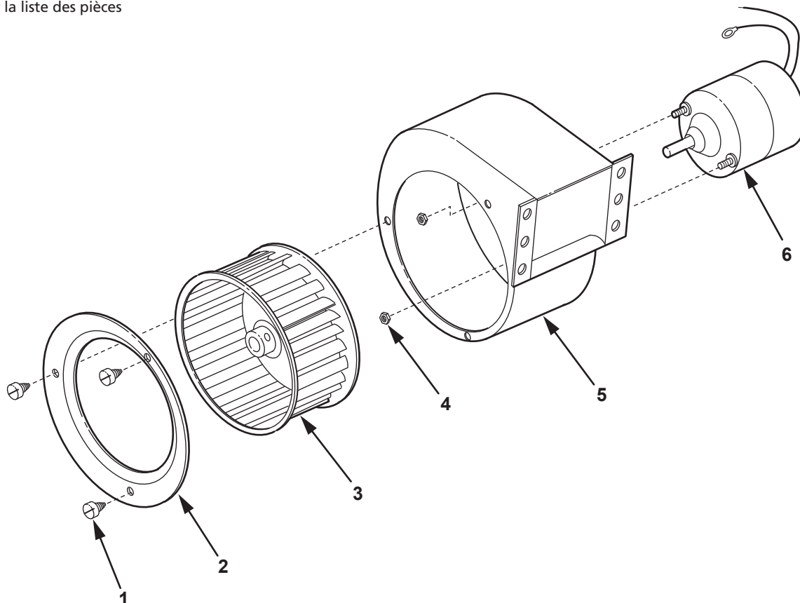
Figure 5 – Illustration des pièces détachées pour Soufflantes
