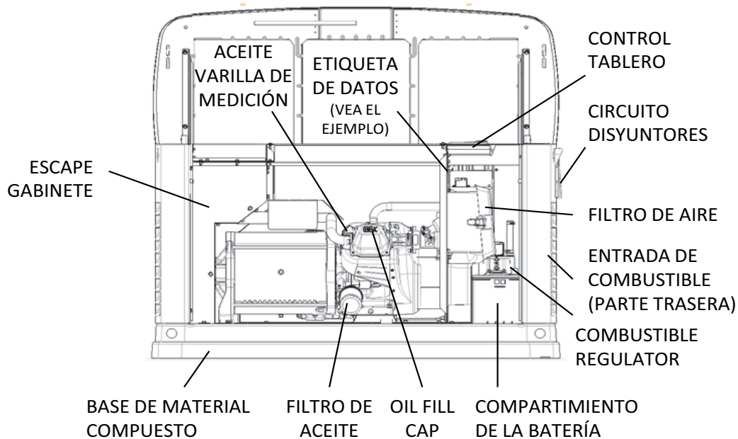
Figura 2-1: Unidad GH-410 motor de 8 kW
