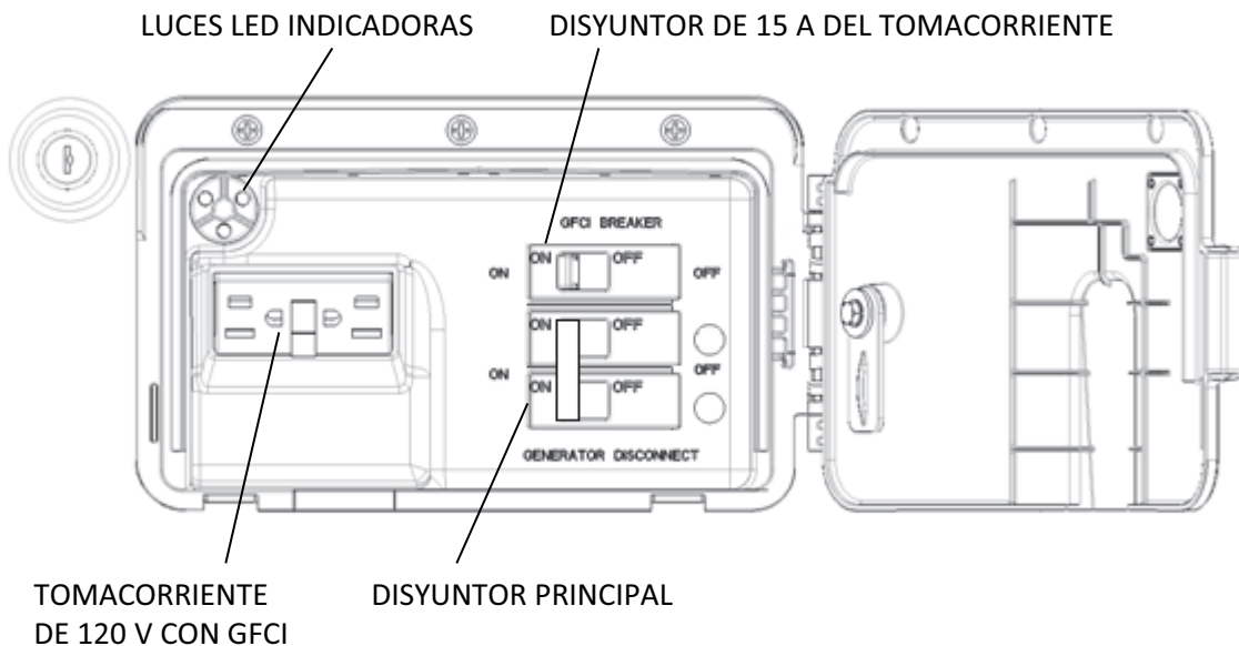
Figura 3-5: Compartimiento lateral abierto
