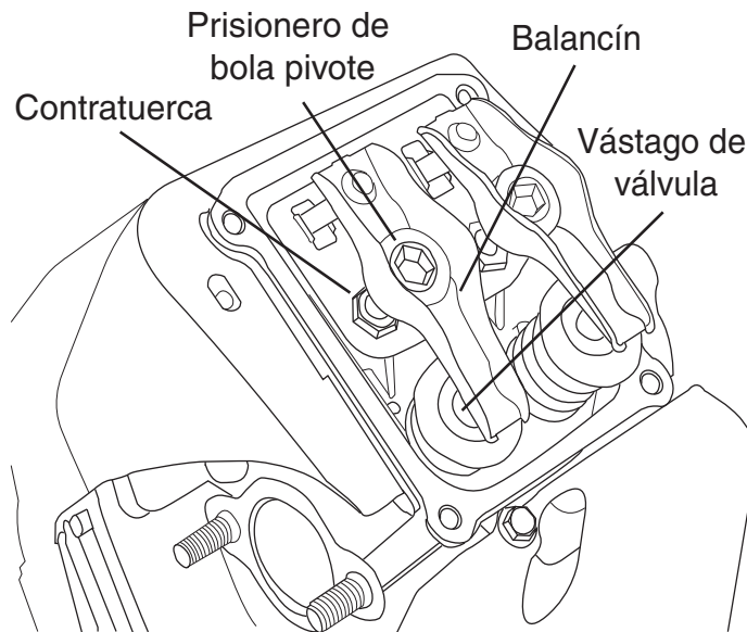
Figura 4-4: Ajuste de la luz de válvulas
