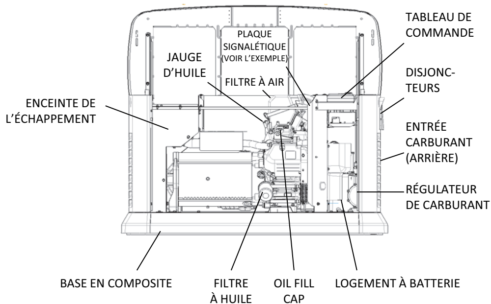
Figure 2-3 : Moteurs GT-990/GT-999, appareils de 13 à 20 kW
