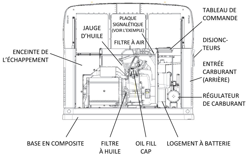
Figure 2-2 : Moteur GH-530, appareil de 11 kW
