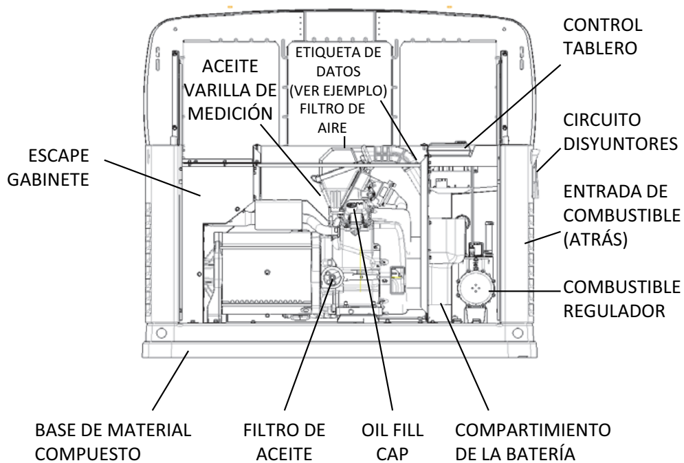
Figura 2-2: Unidad GH-530 motor de 11 kW
