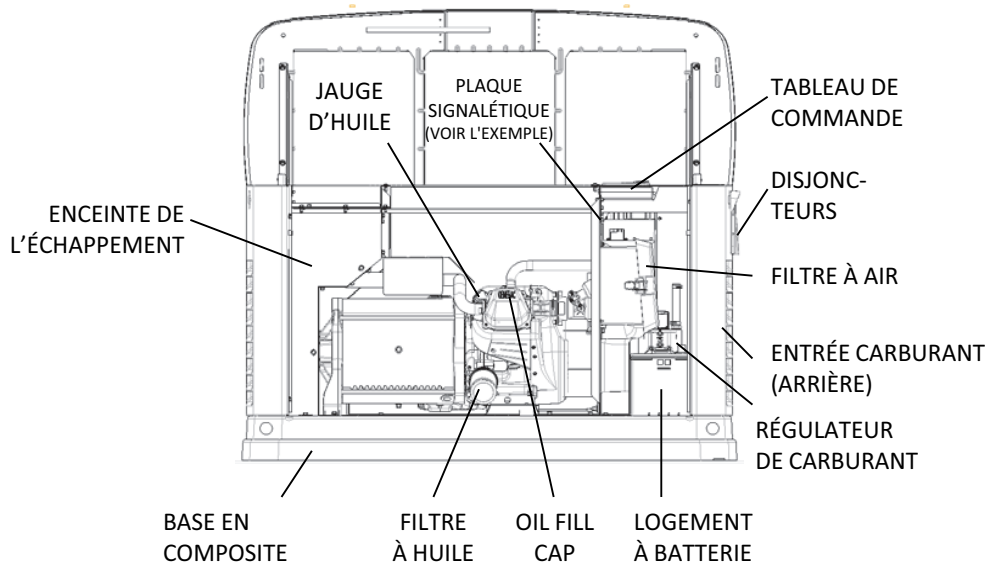
Figure 2-1 : Moteur GH-410, appareil de 8 kW
