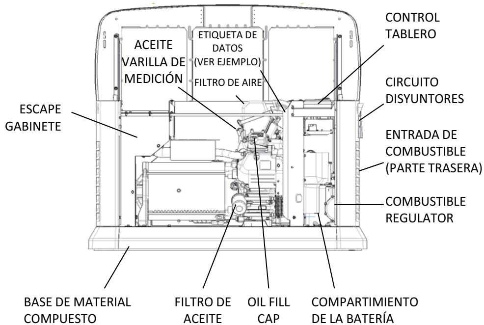
Figura 2-3: Unidad GT-990/GT-999 motores de 13-20 kW
