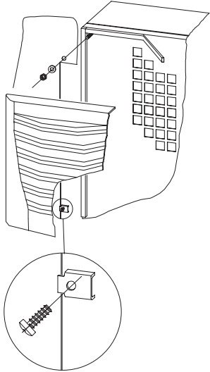
Einbau Internal mounting Montage encastré Inbouw Inbyggnad Incassato Montaje interior
