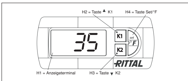
Abb. 6.1 Elektronische Regelung
