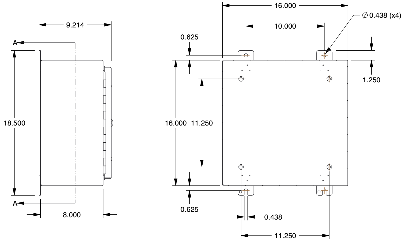
SECTION A-A
